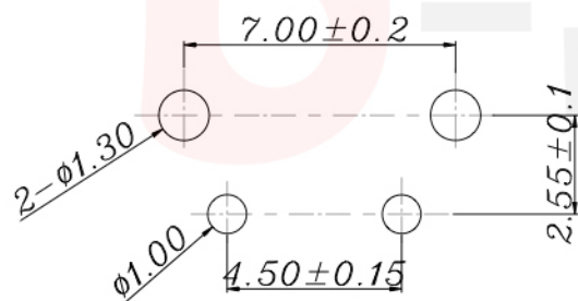
P.C.B LAND DIMENSION
