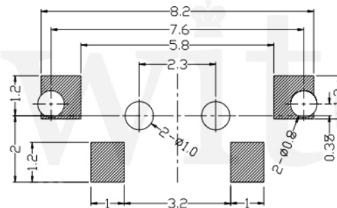
P.C.B LAND DIMENSION
