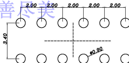
安装图PLERING PLAN
